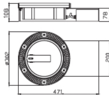
B: 分体式尺寸图
